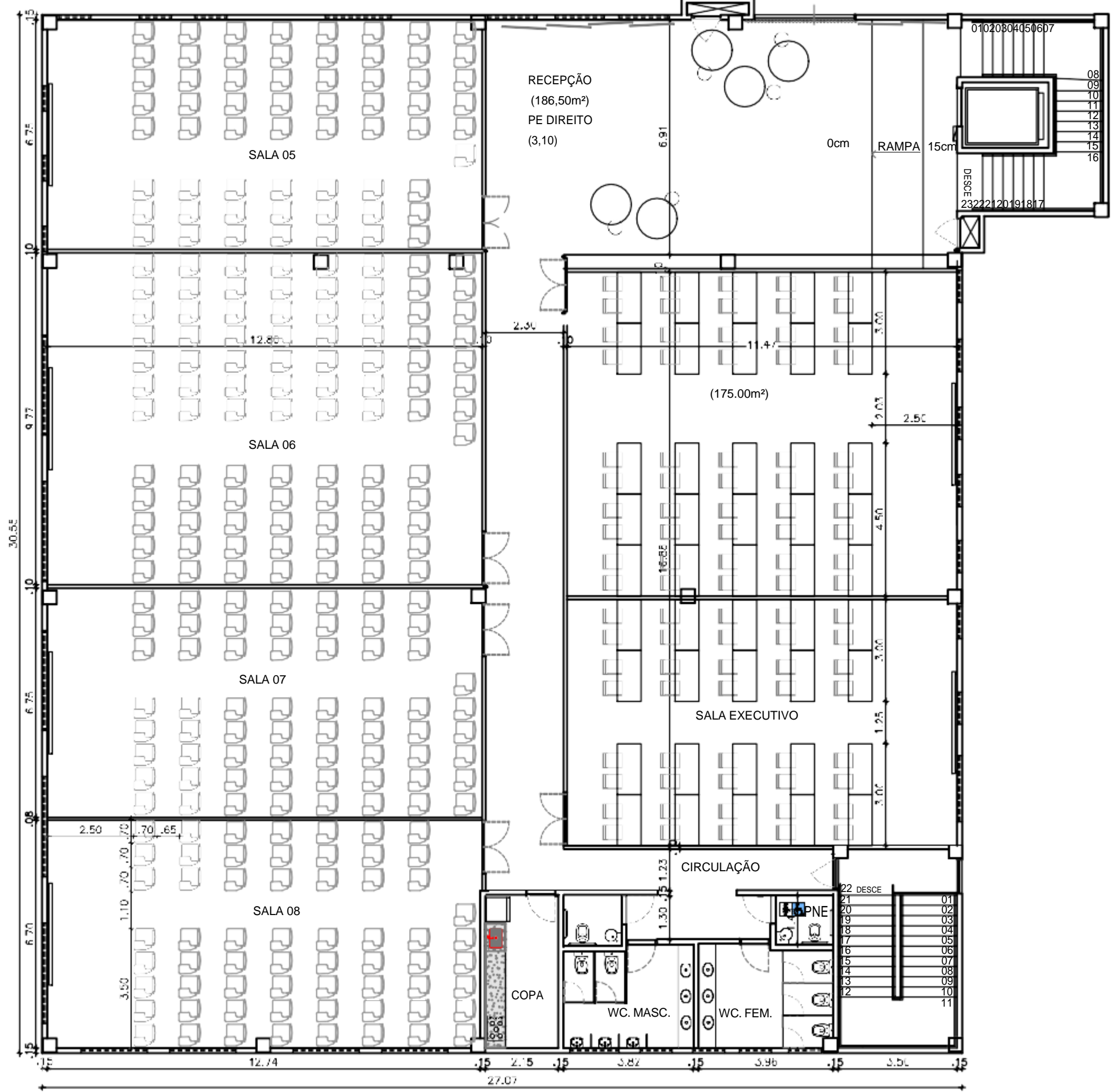
PLANTA BAIXA escala 1/125
